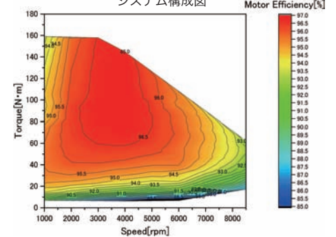
モータ効率マップ
