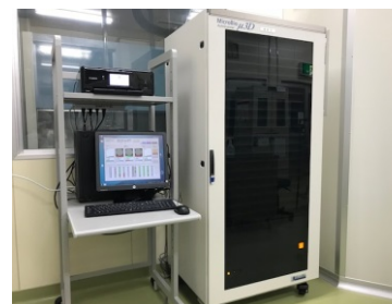
無菌試験迅速測定装置 マイクロバイオμ3D
