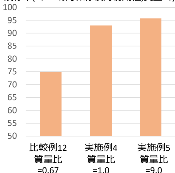
<プロトパキサジオール>
