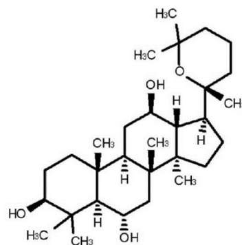
構造式（1） パナキサトリオール
